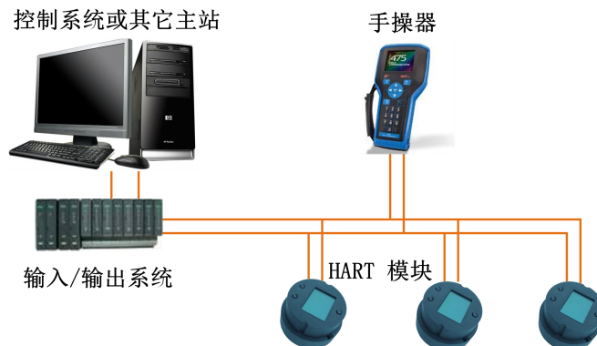
图 7 MS0210 HART 温度套卡组网模式
