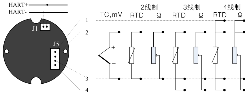
图 4 MS0210 HART 温度套卡接线示意图
